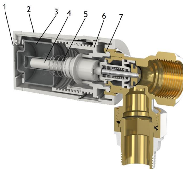
Рис. 2. Устройство термостатической головки TC-S3
