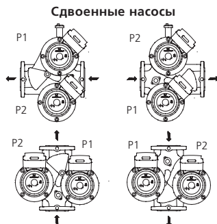
Сдвоенные насосы
