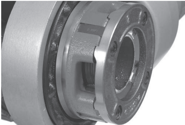
Рис. 15 – Торец трубы ровнен с кромкой резьбонарезных гребенок
