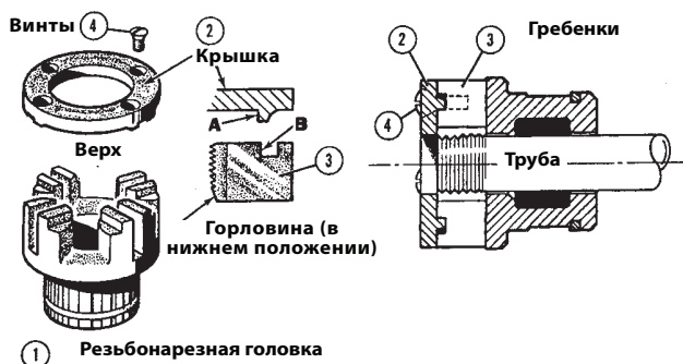
Рис. 17 – Установка гребенок в резьбонарезную головку
