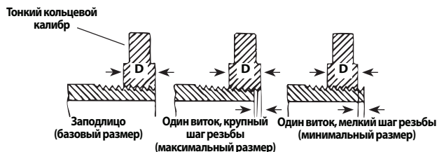
Рис. 16 – Проверка размера резьбы
