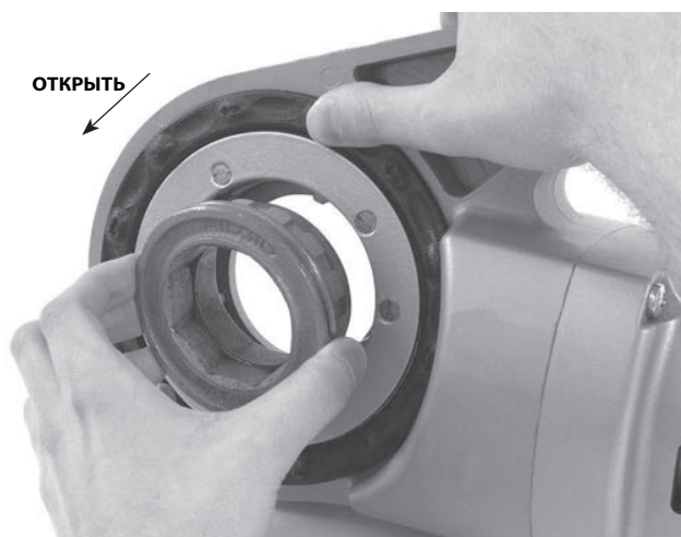
Рис. 8 – Установка переходника в силовой привод 690-I
