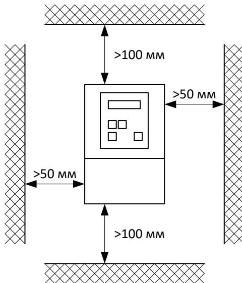
Рисунок 3 – Установка ПЧ
