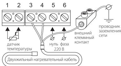
Схема подключения к 3-х проводной электрической сети
