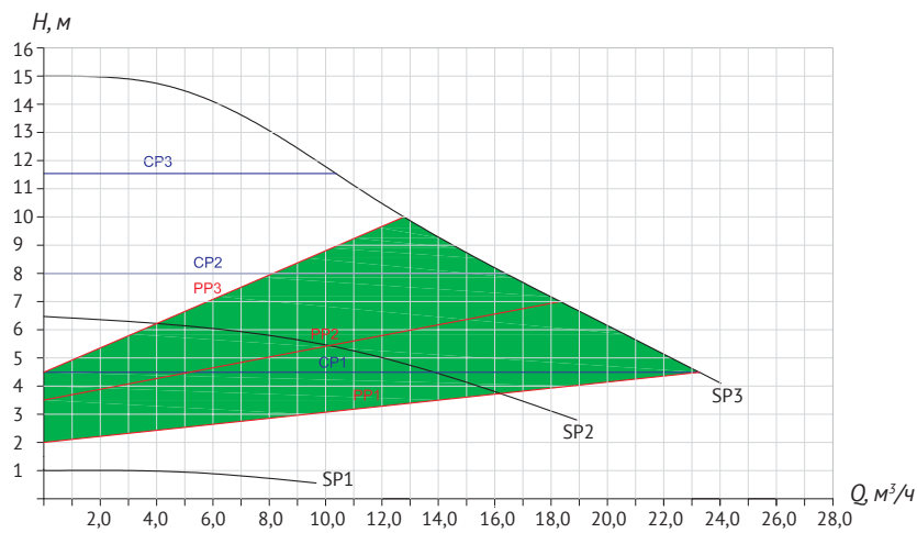
PFE 50-150 280
