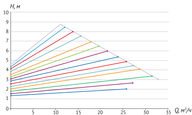
PFE 65-100 340
