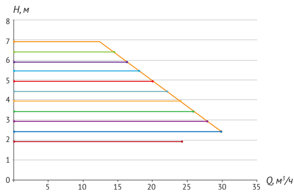
PFE 65-80 340
