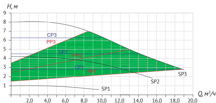
PFE 50-120 280
