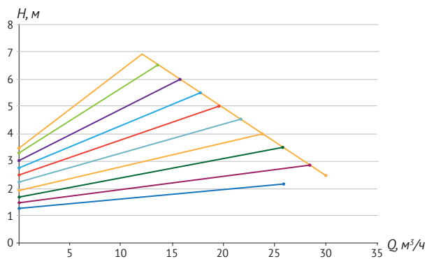
PFE 65-100 340
