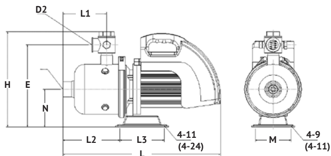
Рисунок 1 – Габаритные и присоединительные размеры
