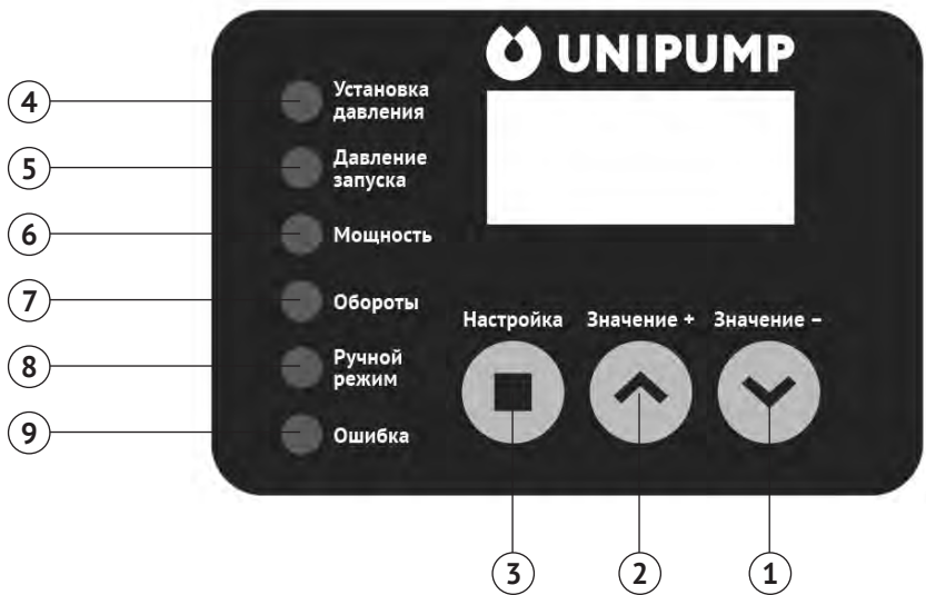
Рисунок 6 – Панель управления
