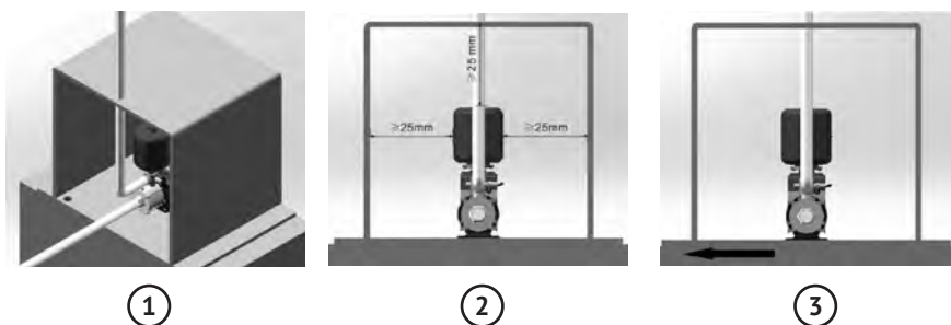
Рисунок 4 – Место установки
