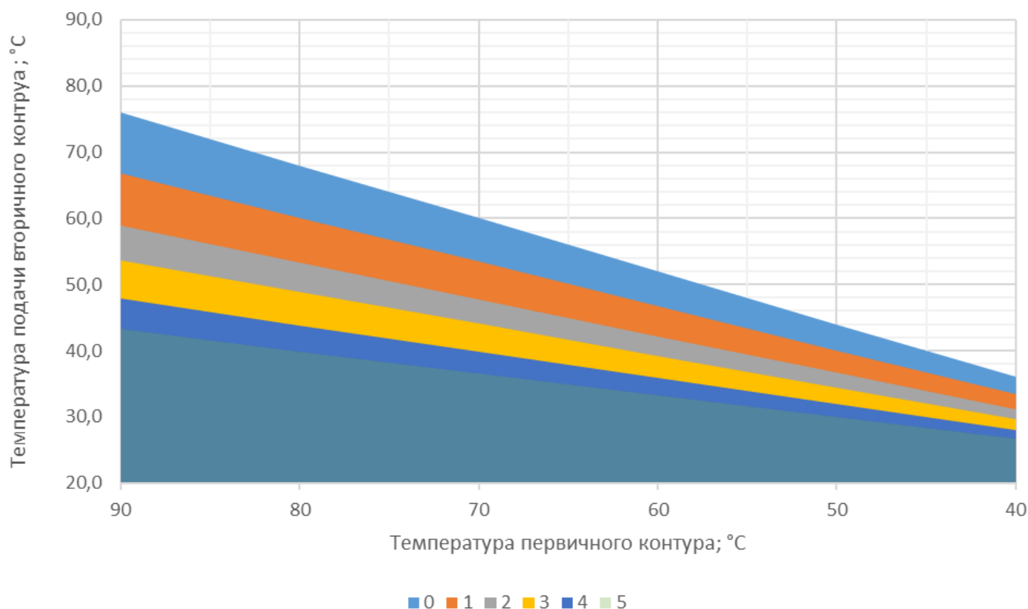
График настройки смесительного клапана
