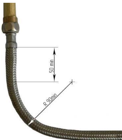
Рис. 3. Требования к монтажу гибких шлангов
