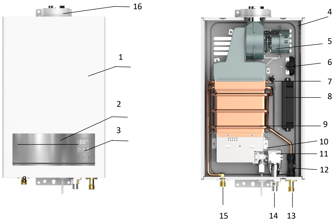
Рис. 2. Аппарат водонагревательный проточный газовый бытовой S12FT
