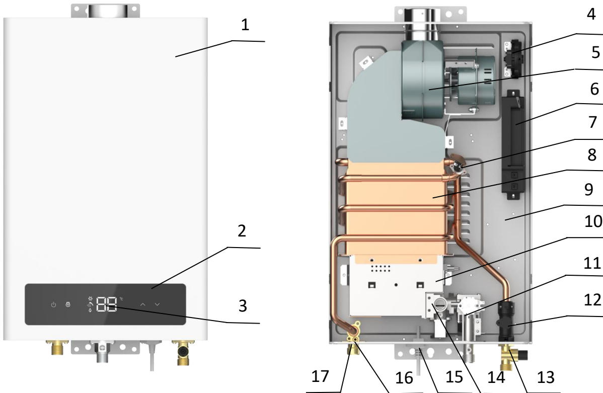
Рис. 1. Аппарат водонагревательный проточный газовый бытовой S13ST, S16ST
